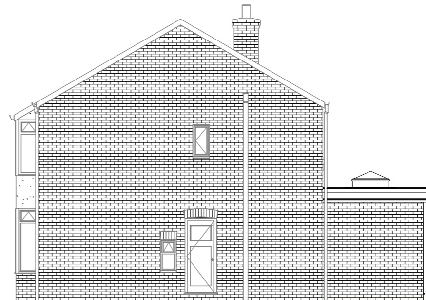
3 Gable 1 : 100
